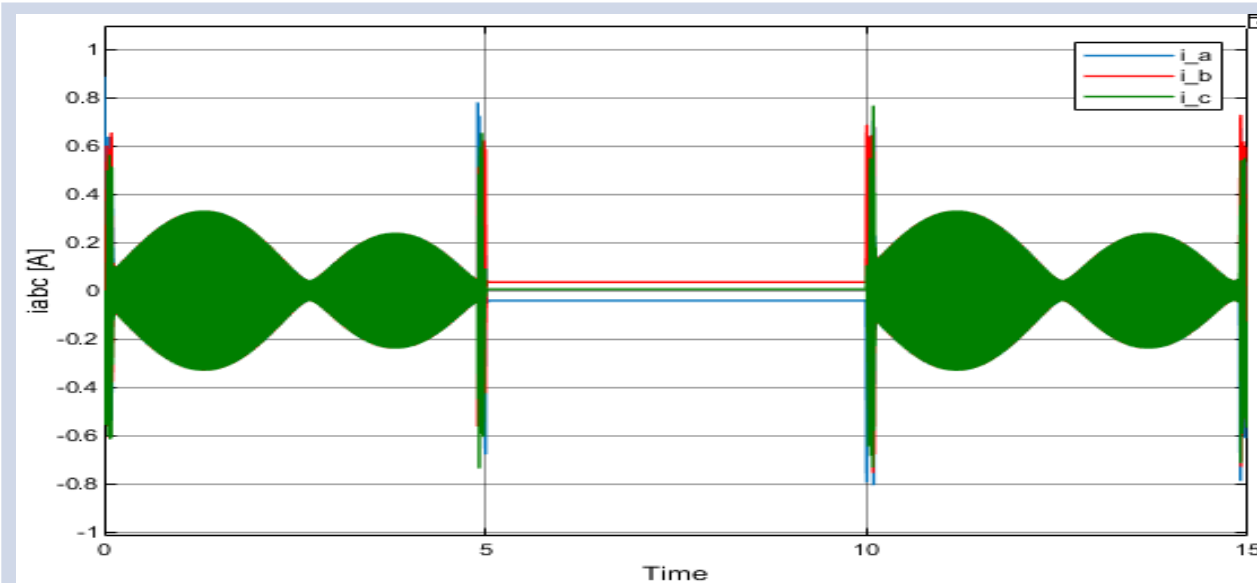
FIGURA: Figura 96: Curvas de corrientes i_{abc} con controlador discreto
