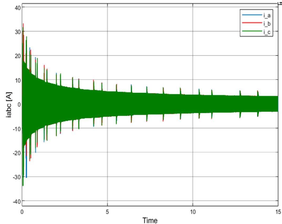
FIGURA: Figura 86— Curvas de i_{abc} con \omega_{n\_modulador} = 6000 \text{ rad/s}
