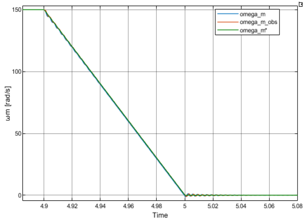
FIGURA: Figura 72— Curvas de velocidad con \omega_{n\_pos} = 4000 rad/s
