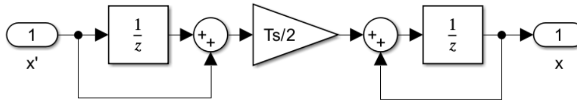
FIGURA: Figura 89— Integrador por trapecios
