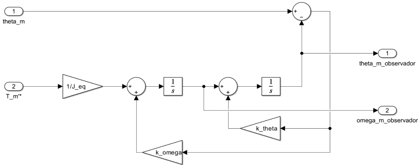
FIGURA: Figura 38— Observador de estado de orden reducido
